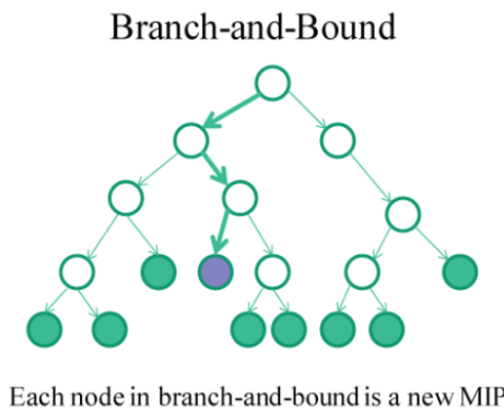
Figura 1 – Cada nó em uma árvore do branch-and-bound é um novo MIP Fonte: (MIXED-INTEGER..., s.d)
