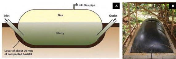
Figura 4 – A) Visão esquemática do biodigestor Balão; B) Biodigestor Balão
