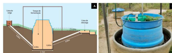
Figura 3 – A) Visão esquemática do biodigestor Sertanejo; B) Biodigestor Sertanejo.
